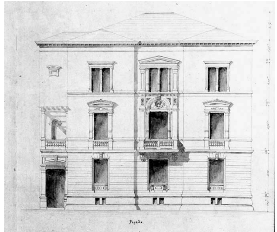
Fassadenentwurf für das Haus Bahnhofstraße 27 in Heilbronn; 1874.
